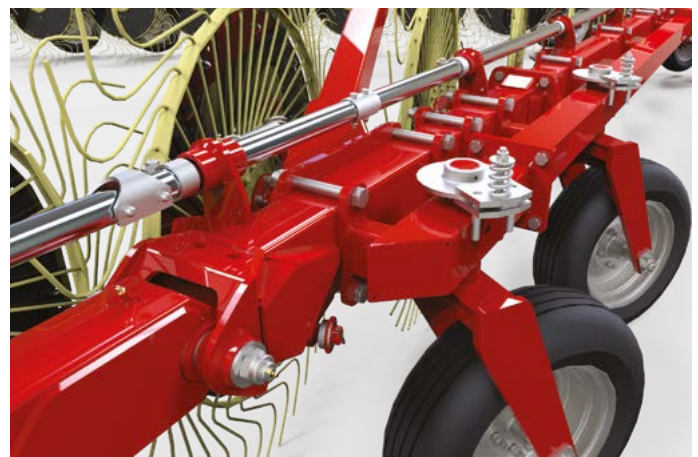
Reinforced structure on the models ERS 18, 20 and 22. The double tubular guarantees an excellent strength and flexibility to the frame. Structure renforcée modèles ERS 18, 20 et 22. Le double tubulaire garantit au châssis une excellente résistance et flexibilité.
